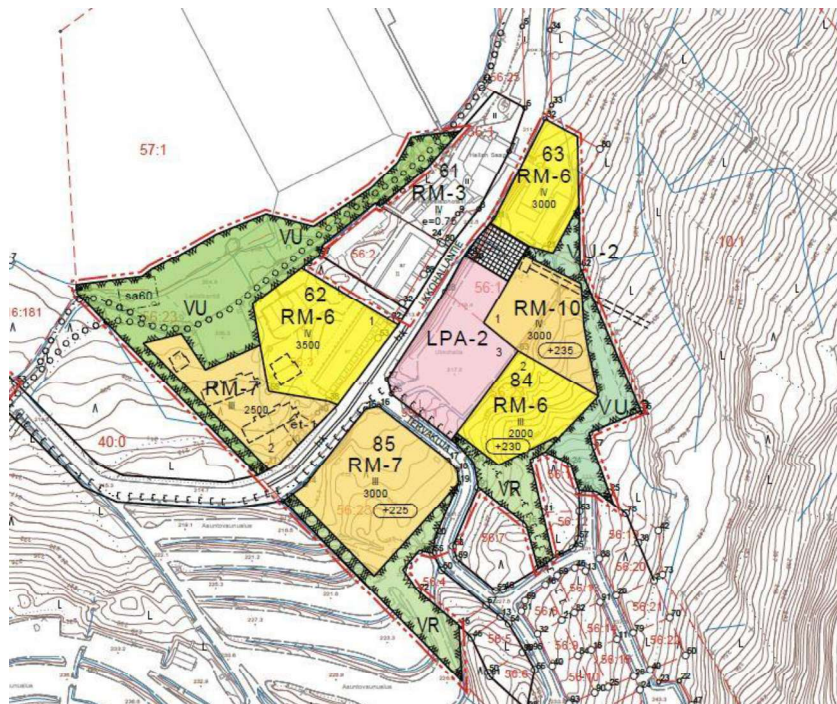
Kuva 21 Kunnanvaltuuston 14.11.2017 hyväksymä muutos
